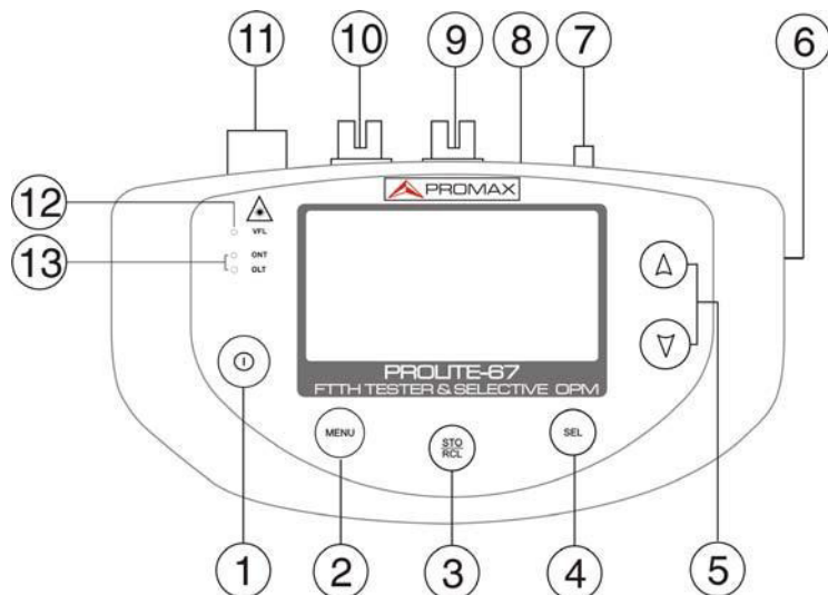
Figura 2.- Vista frontal.
