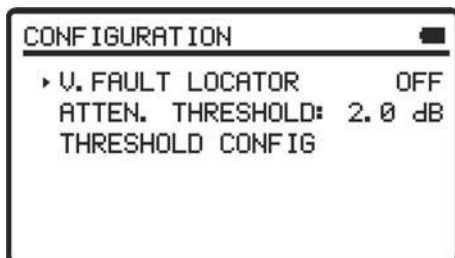
Figure 5.- Écran CONFIGURATION.
